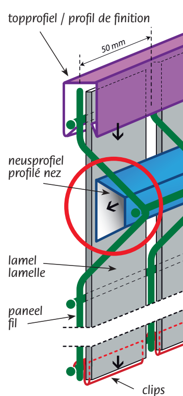
Trapezium-neusprofiel Profilé-nez
